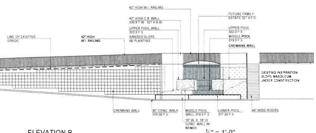
ELEVATION B
