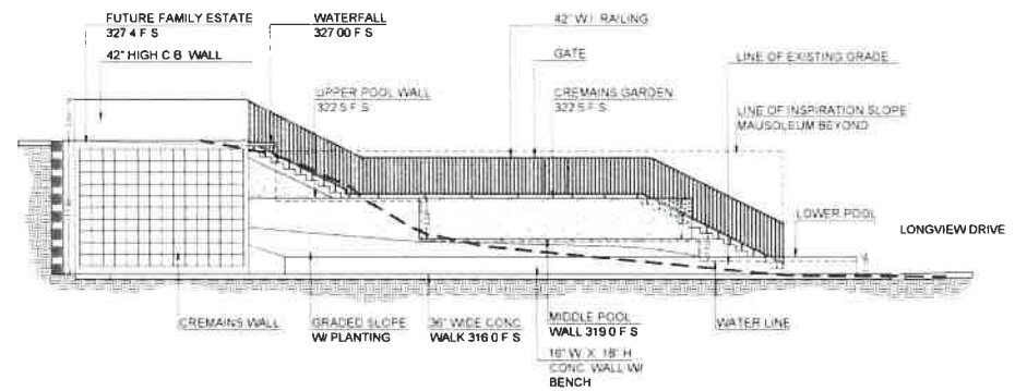
ELEVATION A
