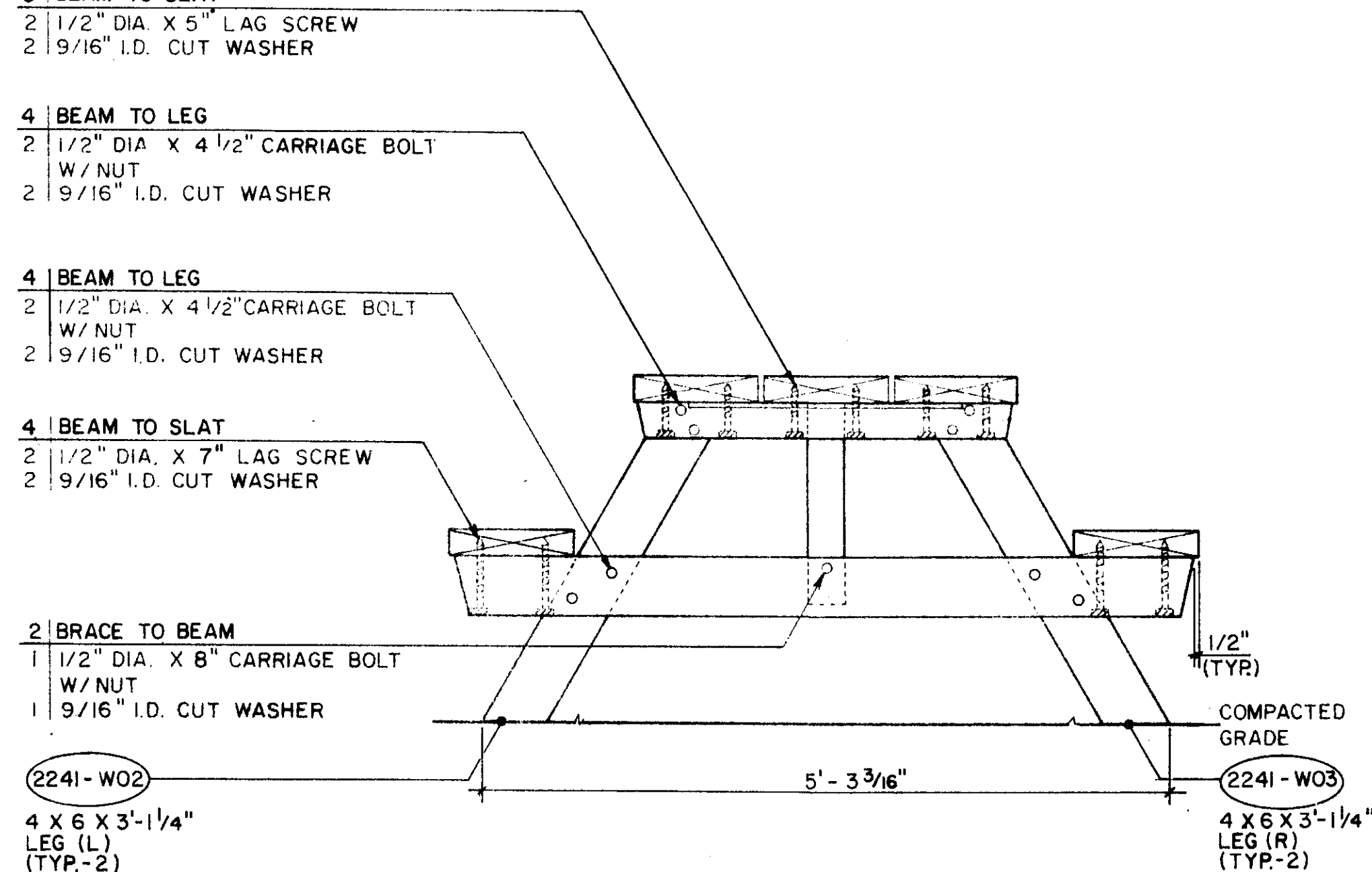
ELEVATION
